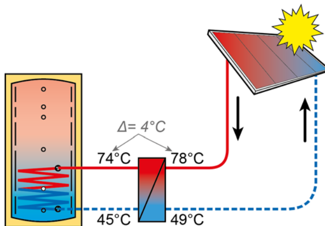
Sl. 7-110: Princip regulacije
