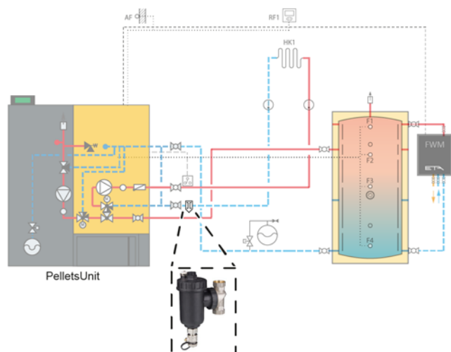
Sl. 8-2: Vgradni položaj pri kotlu z integriranim ogrevalnim krogom
